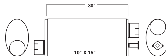
MODEL: CAT 988B 7W8445
